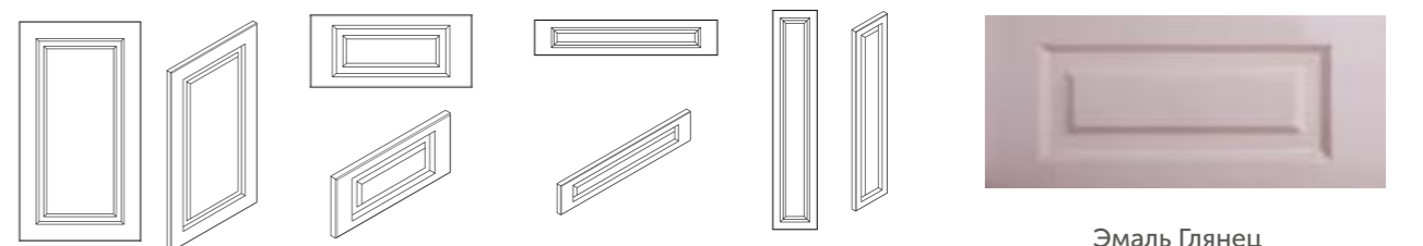
Фасад с филёнкой, прямой Шувлядка 177 Шувлядка 116 Накладка 716*147
