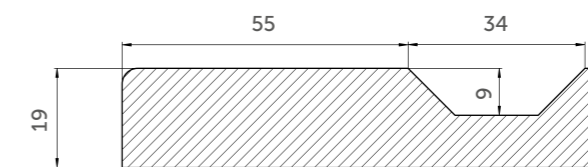
Сечение профиля
